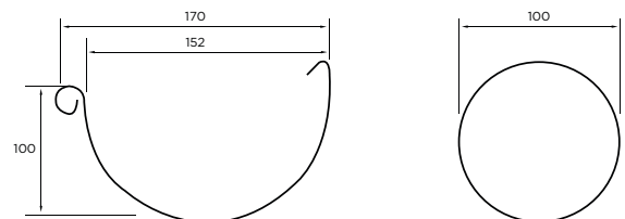
Regenwaterafvoersysteem 165/100 mm
